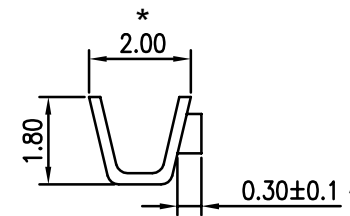
D-D SECTION
