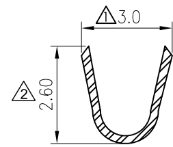
A-A SECTION
