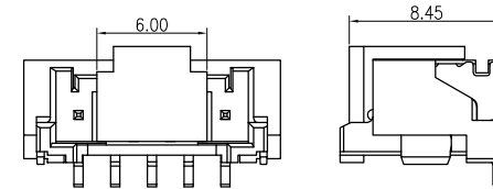
加盖示意图
