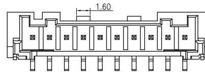
10-15P两个卡扣 视图
