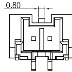
2P 视图
