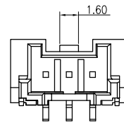
3P 视图
