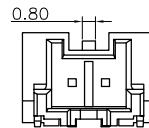
2P 视图
