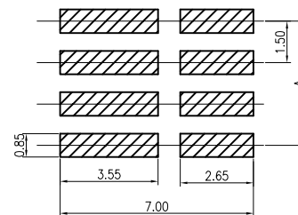
P.C.Board Layout
